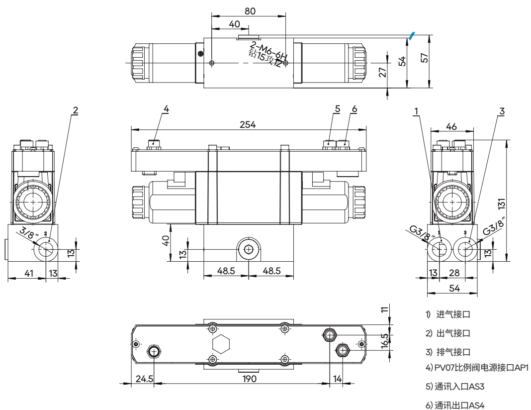
尺寸图
