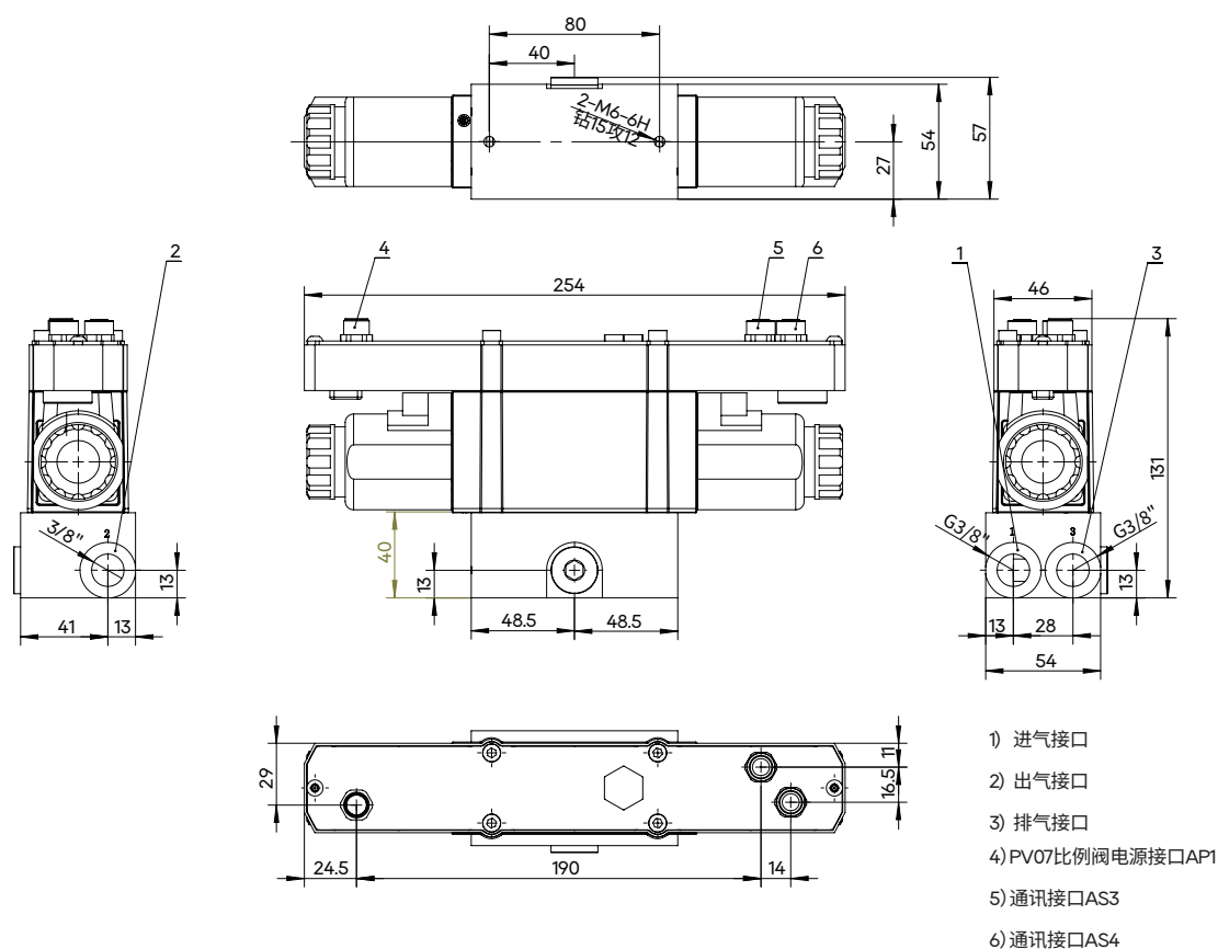
尺寸图
