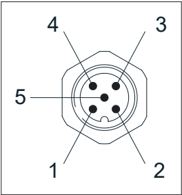
AP1 插头 - M12 - 5针
