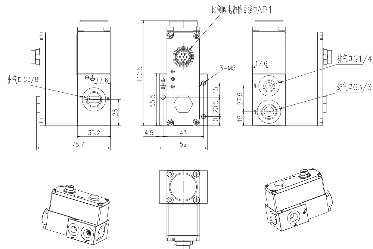
尺寸图
