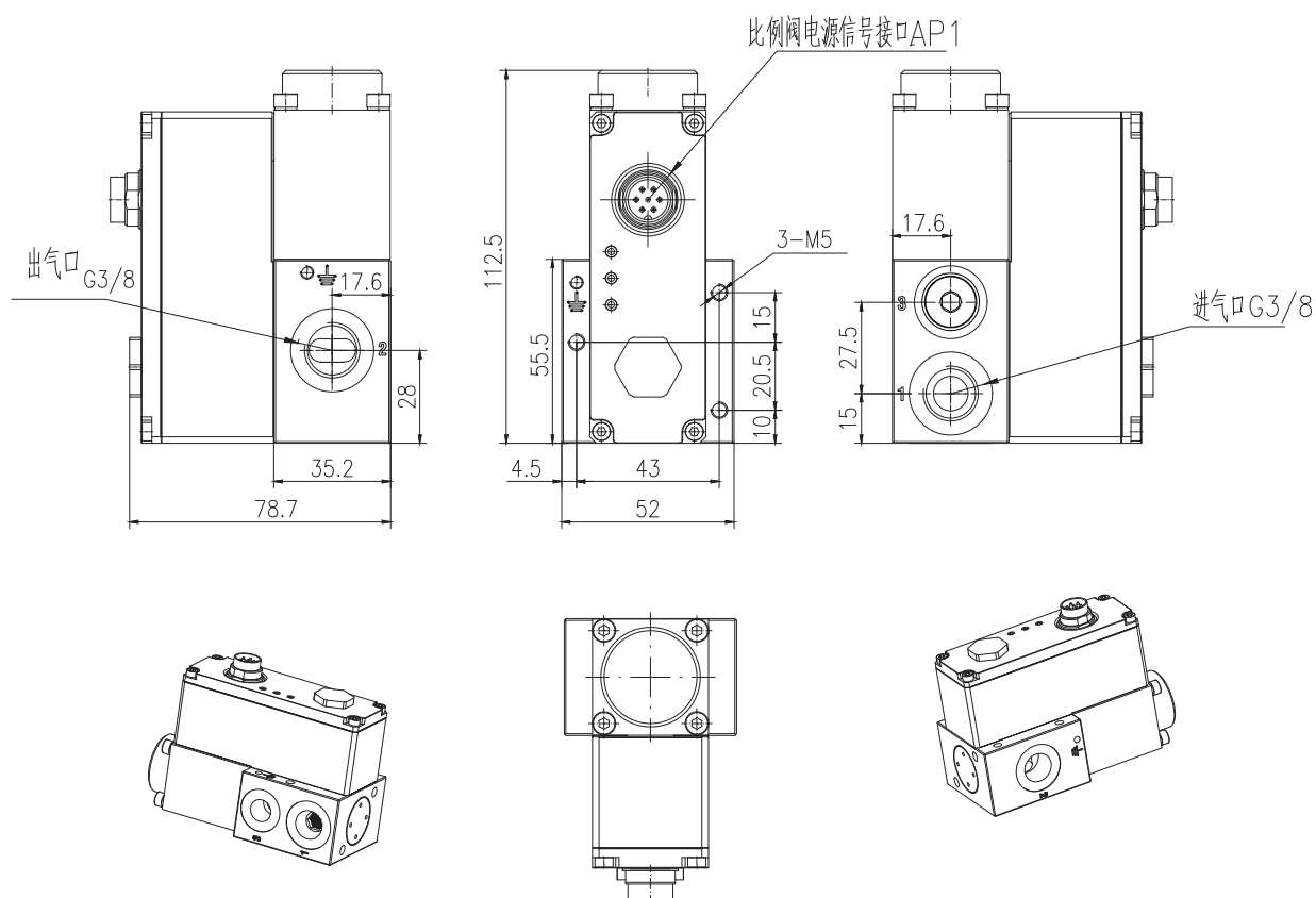
尺寸图
