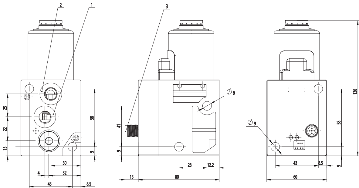
尺寸图
