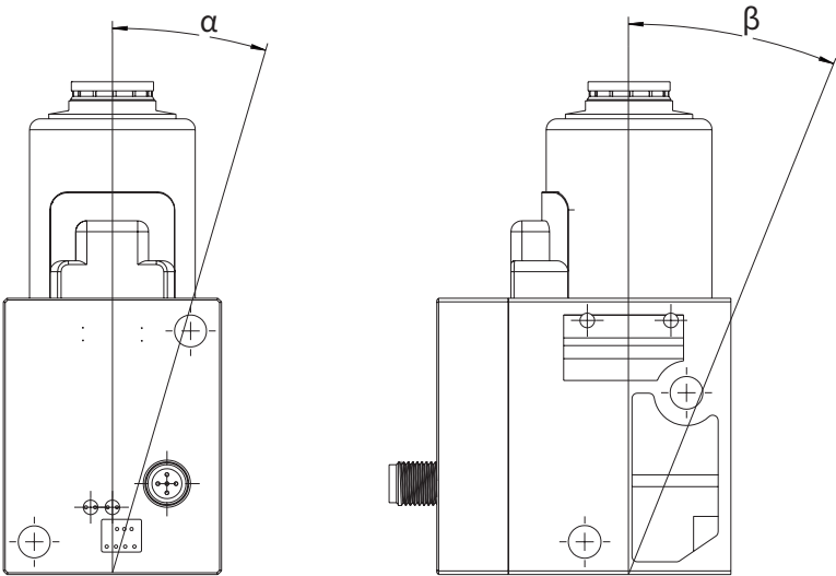
安装角度应符合以下要求：α=±90° β=0°-90°
