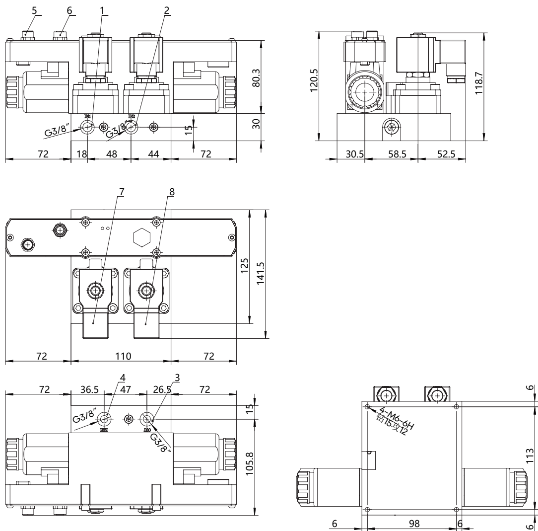
尺寸图
